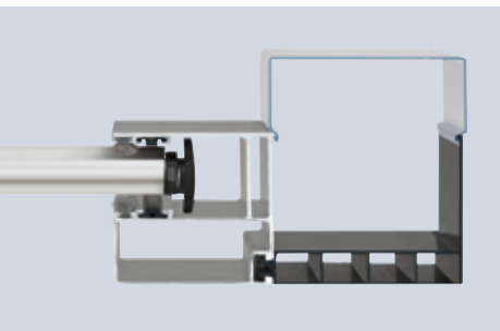
Rideau à lames SB / TGT, profilé Decotherm S, avec crochet anti-tempête synthétique
