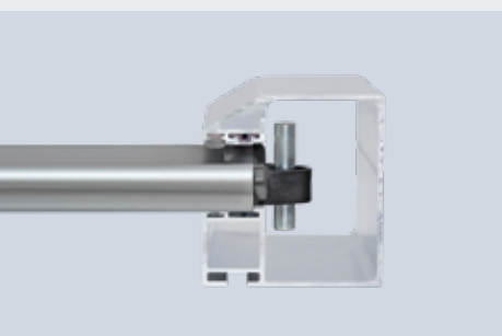
Rideau à lames DD, profilé Decotherm S, avec crochet anti-tempête en acier (à partir de 7 500 mm de largeur et/ou de hauteur ou, en option, à partir d'une exigence de charge au vent plus élevée)
