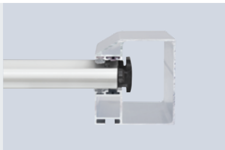
Rideau à lames DD, profilé Decotherm S, avec crochet anti-tempête synthétique
