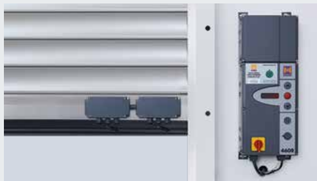
Unité de transmission sans fil Equipement en option pour la transmission des signaux du tablier de porte à la commande via Bluetooth – au lieu d'un câble spiralé. L'alimentation électrique est fournie par une pile puissante. Pour les commandes : 445 R / 460 R
